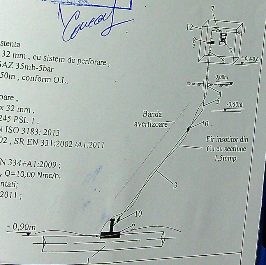
SCHEMA IZOMETRICA RACORD GAZE NATURALE R.P.
